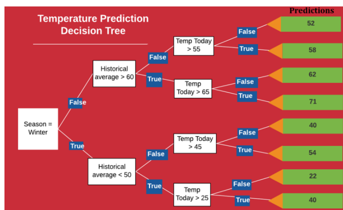
2 paveikslas. Sprendimų medis ( https://medium.com/@williamkoehrsen/random-forest-simple-explanation-377895a60d2d )
