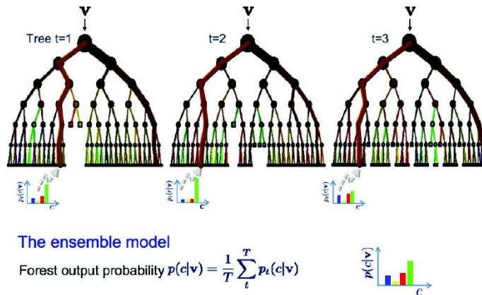
3 paveikslas. Random Forest metodo iliustracija (Leek)
