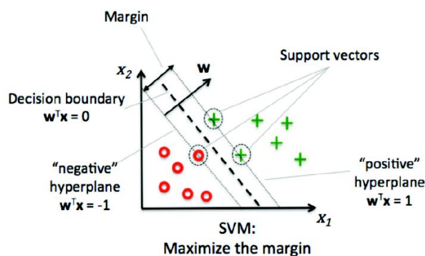
4 paveikslas. SVM metodo iliustracija (Raschka 2016)
